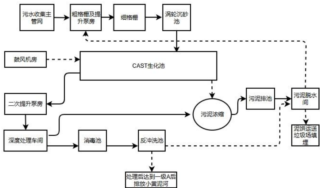
图 4-1 污水厂污水处理工程工艺流程图
